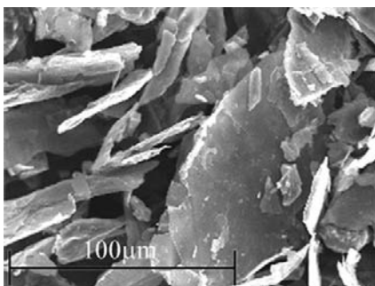
SEM
