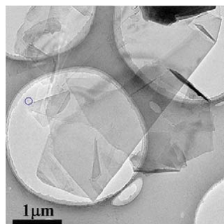
TEM
